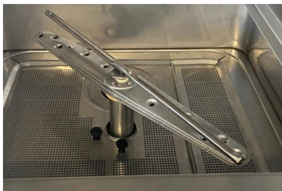
Vaskekammer med spylearm, tankfiltre og låser.
